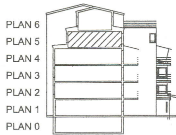
Tvärsektion
