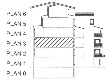
Tvärsektion
